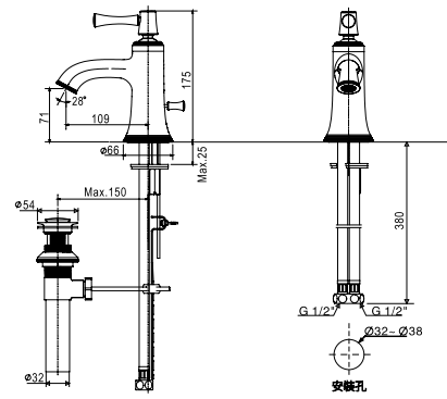
Heritage 面盆龍頭 FFAS0201-101500BCO
